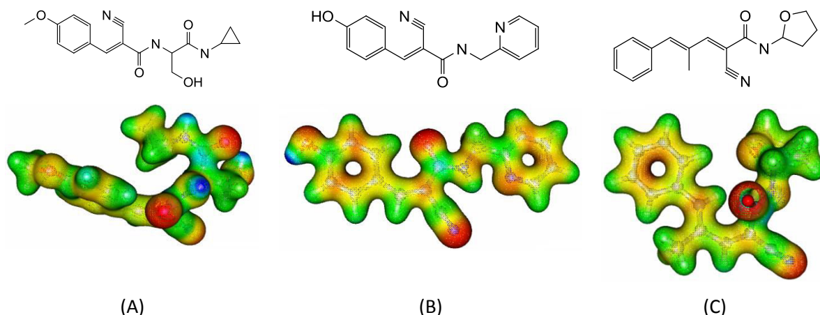
Figura 2. Estruturas e o Mapa do potencial eletrostático dos ligantes 17 (A), 25 (B) e 68 (C)
