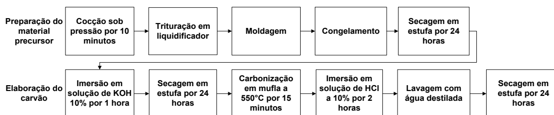
Figura 1. Etapas do processo de elaboração dos briquetes de carvão
