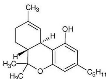
Figura 4. Estrutura química do \Delta^9 -THC
